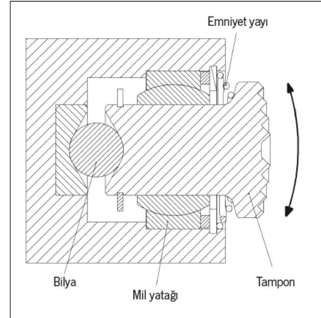
Mil yatağı çalışma diyagramı
