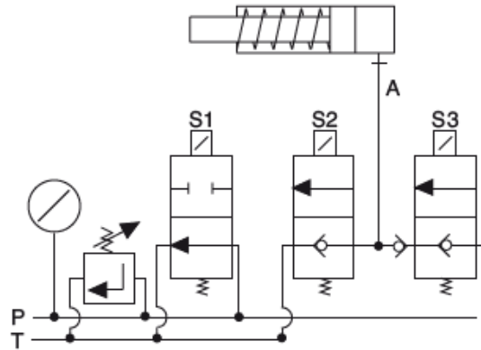
Tek etkili silindirler için VEP-3/3-1 ve VEP-3/3-2
