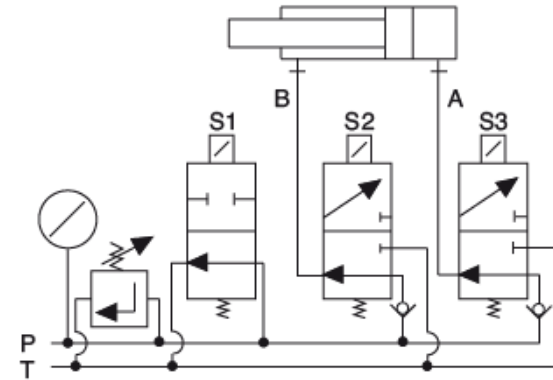
Çift etkili silindirler için VEP-4/3-1 ve VEP-4/3-2
