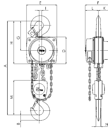
Model Yalelift 360, 5000 kg, çift donam
